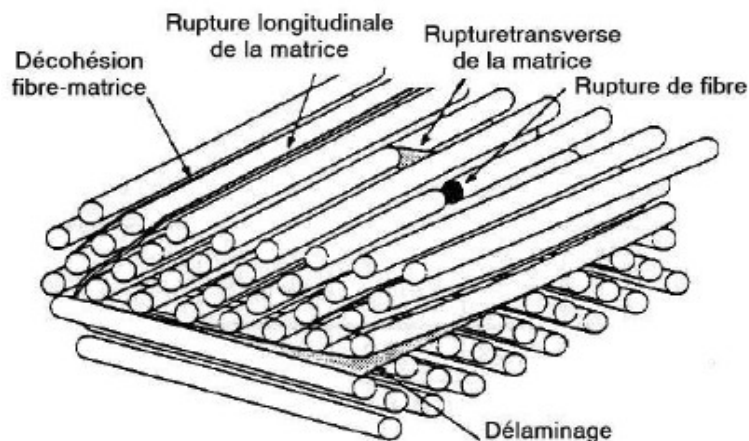
Figure 2. Résumé des différents défauts des matériaux composites à fibres de carbone [7]
